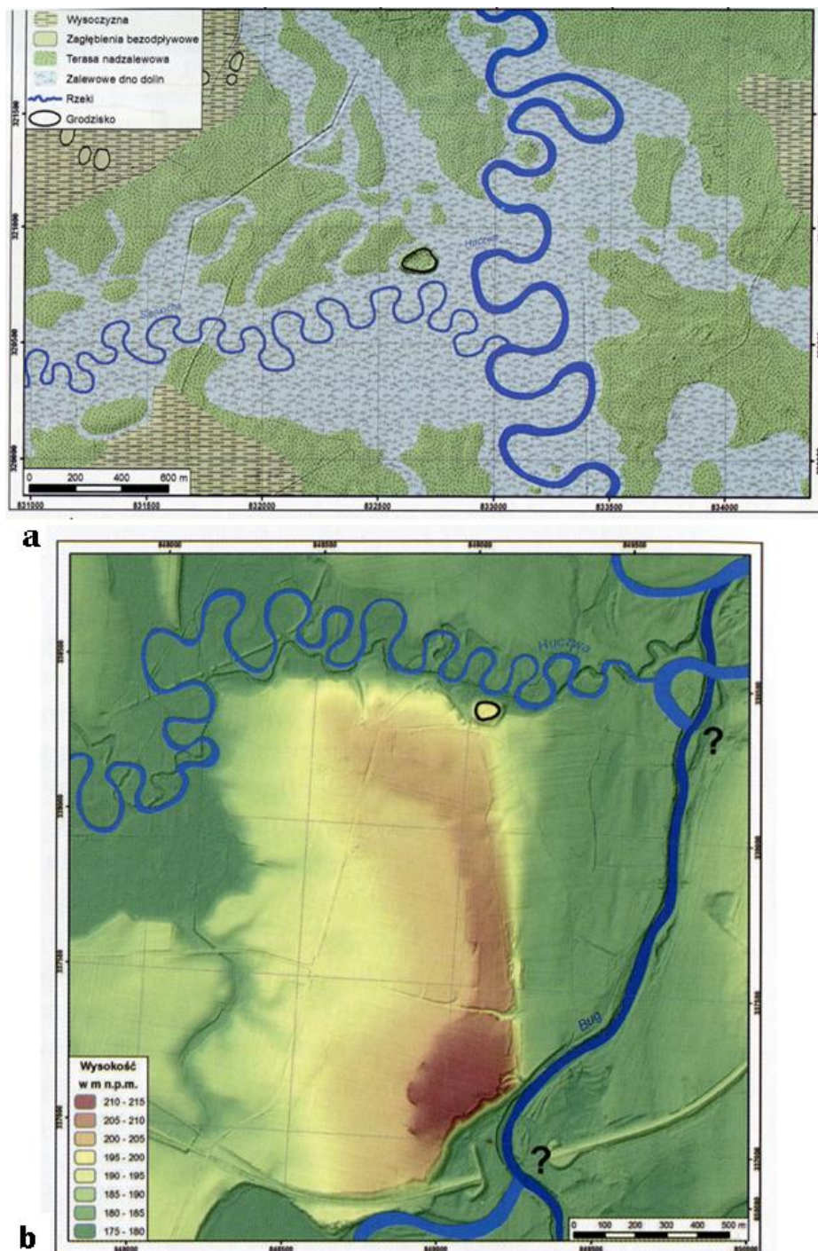
Рис. 10. Зміна русла річки Гучва біля літописного Червена (а) і Волиня (b) (за Reder, Demczuk, 2019) Fig. 10. Change of the riverbed of the Huchva River near annalistic Cherven (a) and Volhyn (b) (by Reder, Demczuk, 2019)
