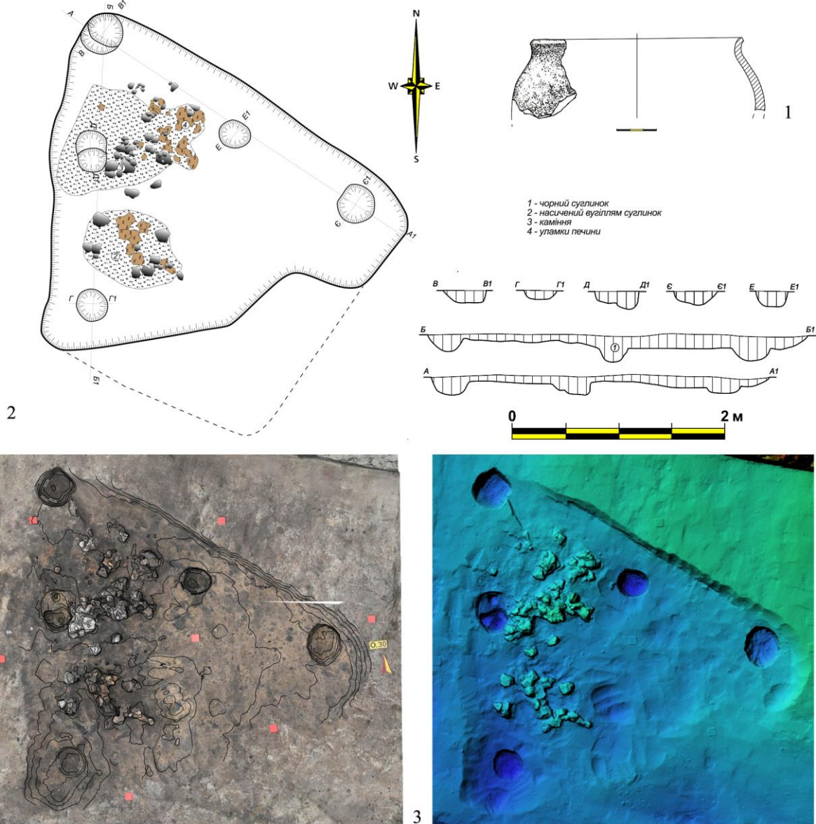
Рис. 10. Поселення Сокульники-1, житло (об'єкт 30) ранньослов'янського часу (VIII–IX ст.): 1 – уламок посудини із заповнення об'єкта; 2 – план і перетини об'єкта; 3 – 3D реконструкції об'єкта (рис. Д. Мостовий, З. Ільчишин, І. Принада)
