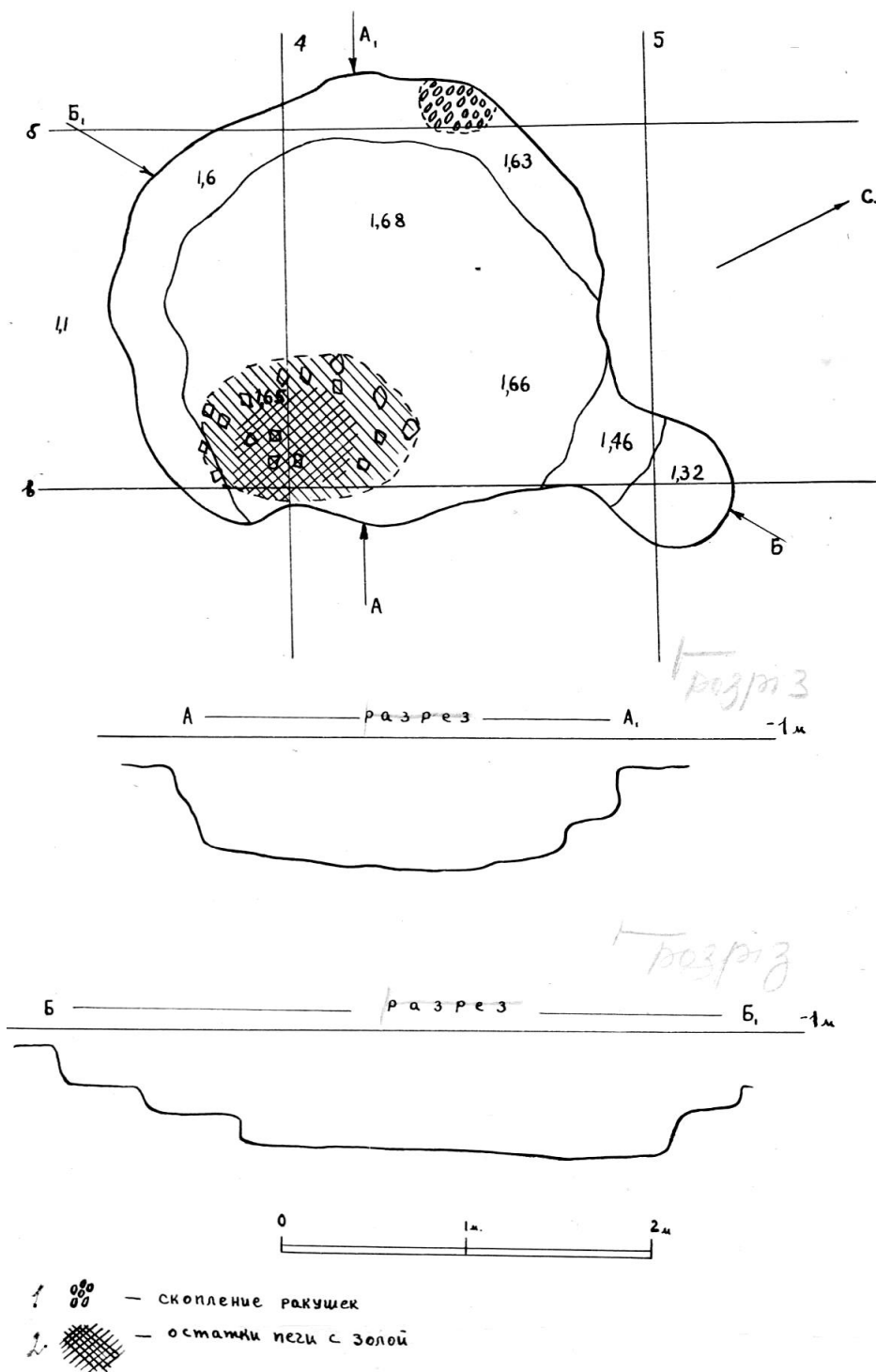
Рис. 4. Перебиківці–Перед Устя. План та перетини напівземлянки скіфського часу
