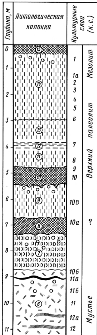
Fig. 3. Molodovo V. Stratigraphic sequence by I. Ivanova (1987; modified by the author) Рис. 3. Молодово V. Стратиграфія за І. Івановою (за Іванова, 1987; з модифікаціями автора)
