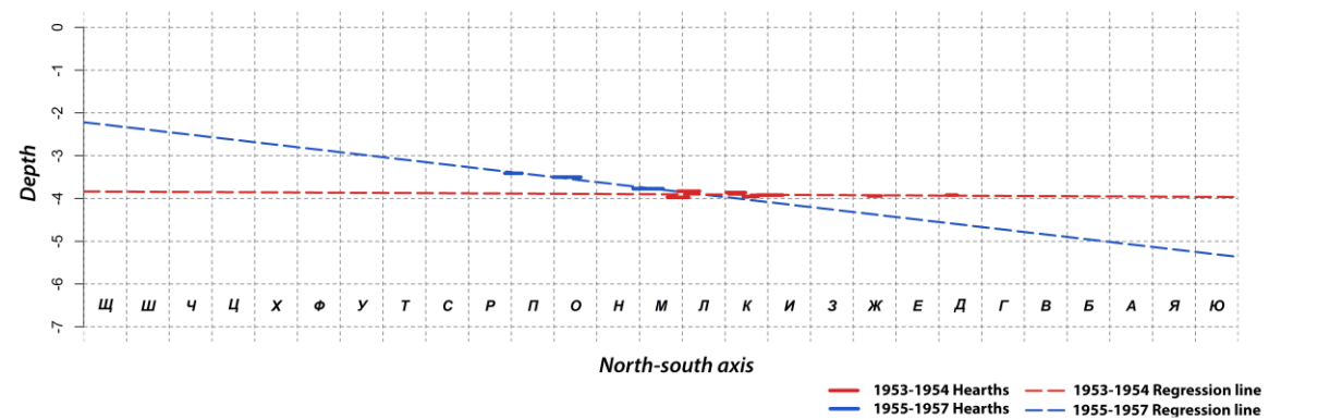
Fig. 25. Molodovo V. Level 8, 1953–1957 hearths and regression lines, side view (from the east) Рис. 25. Молодово V. Культурний шар 8, вогнище та лінії регресії на ділянці розкопу 1953–1957 рр., профіль (вид зі сходу)
